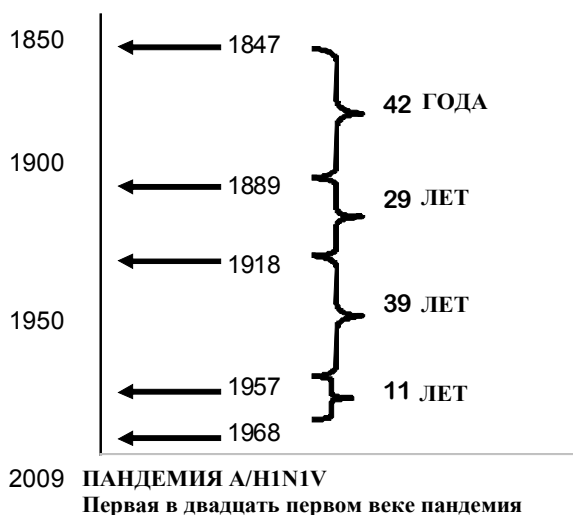
Фигура 4: Частота гриппных пандемий с 1847 года.
